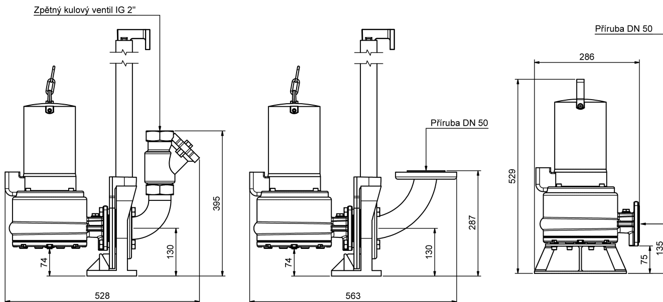
stacionární instalace
